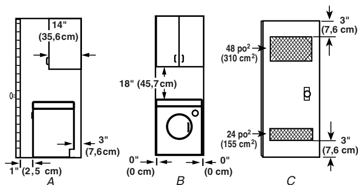
A. Vue latérale - placard ou endroit exigu B. Encastrement C. Porte de placard avec ouvertures d'entrée d'air
